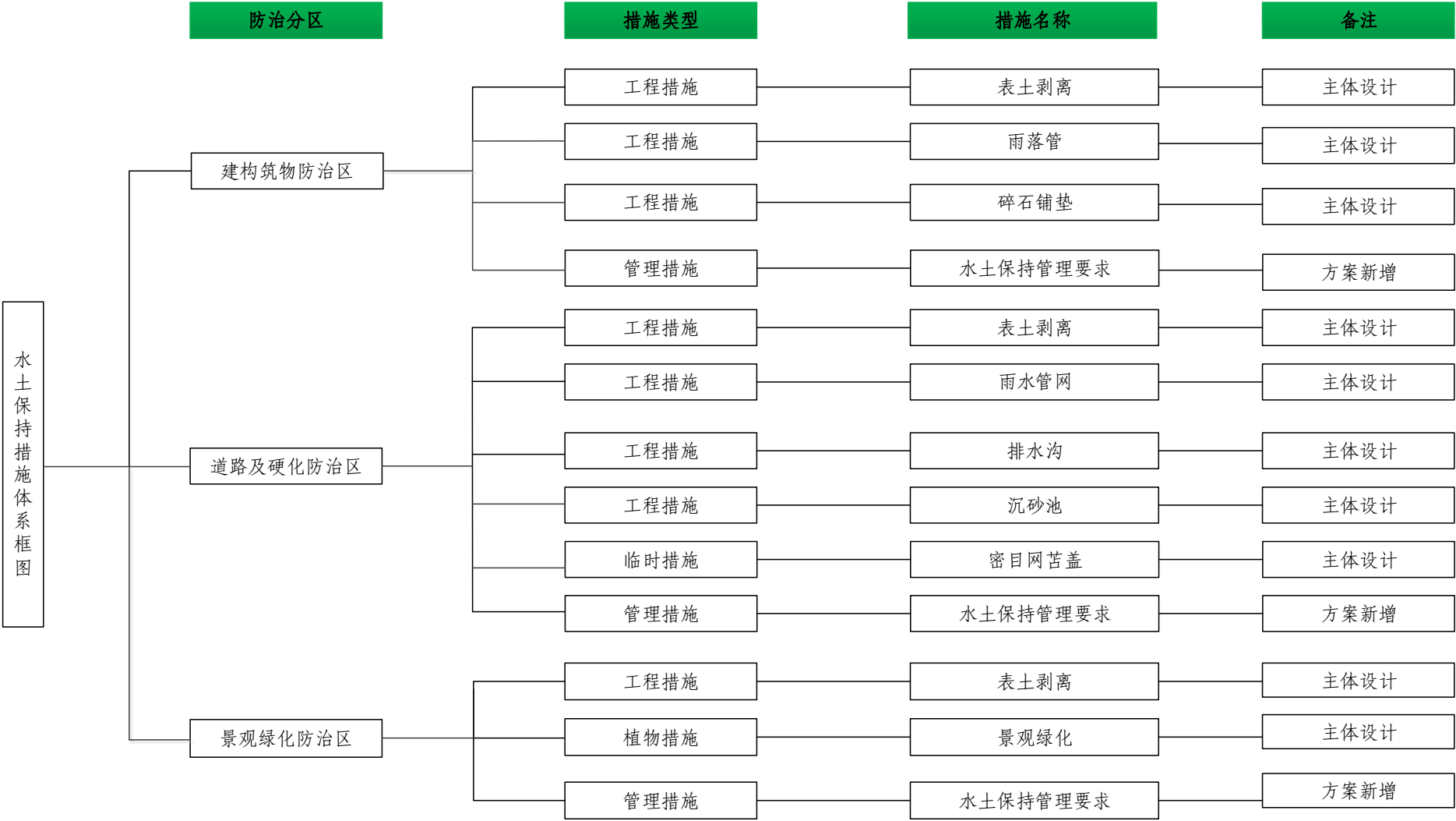
图 5-2 水土流失防治措施体系框图
