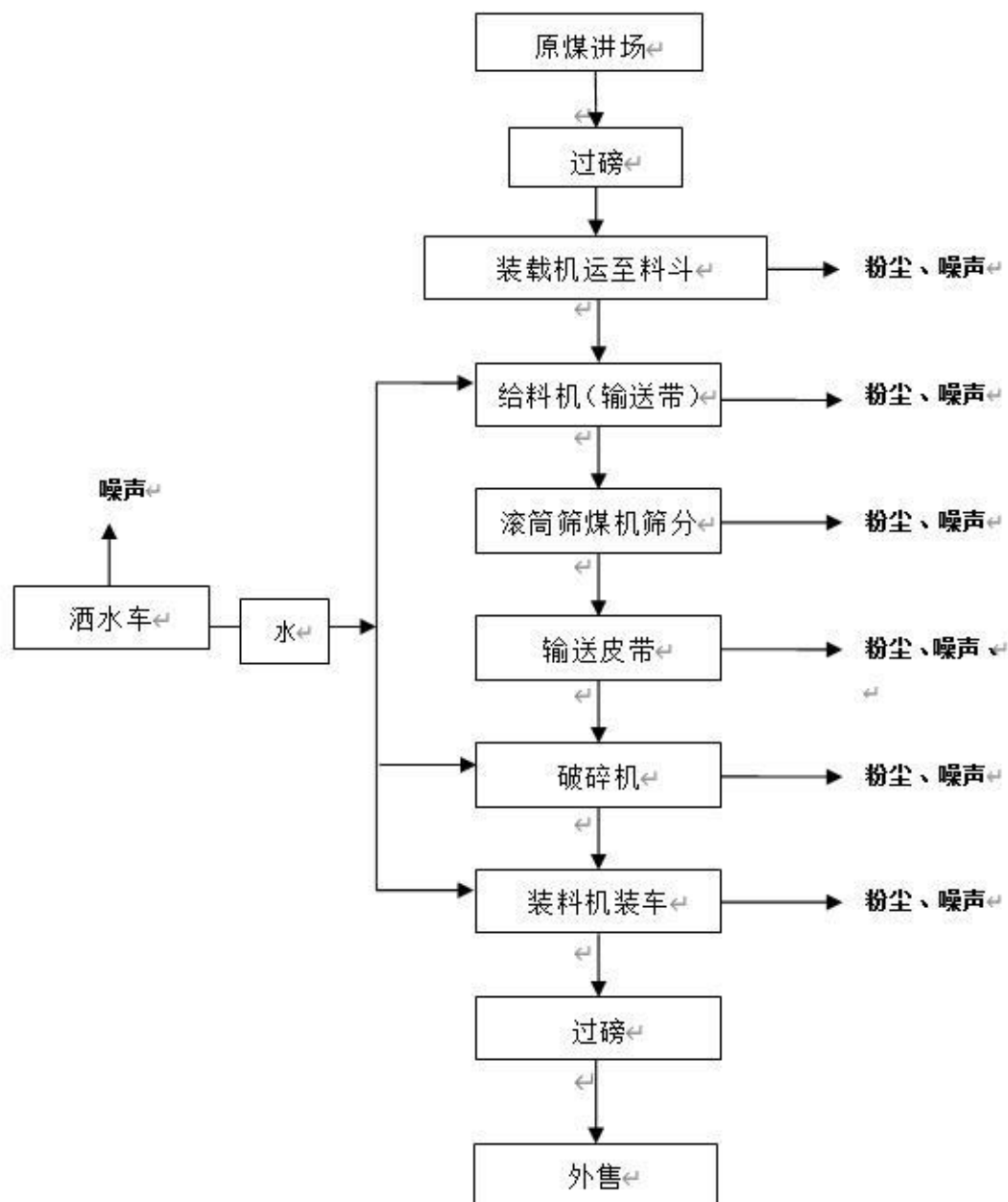
图 2-4 运营期生产工艺流程
