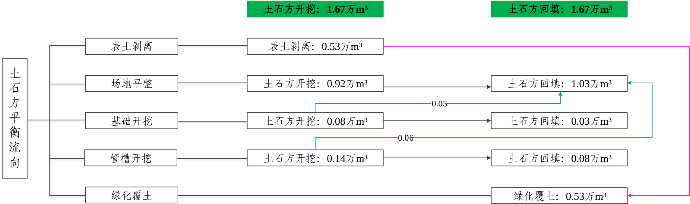
图 2-5 工程土石方平衡及流向图
