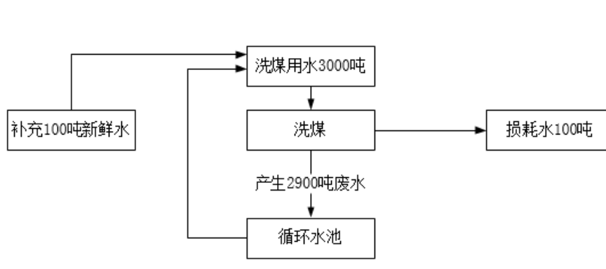
图 2—3 水平衡图
